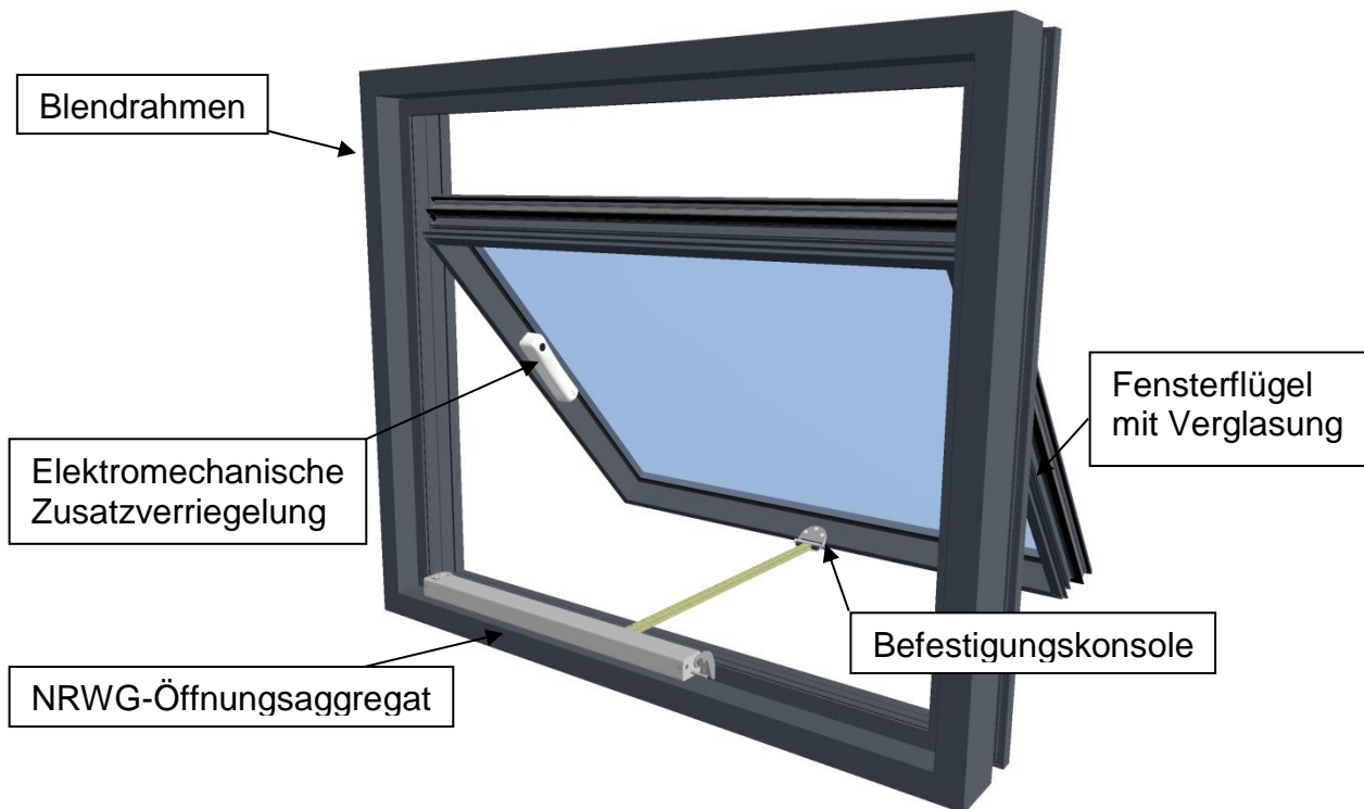
Bild 3: Beispielhafte Darstellung für ein in ein Fenster integriertes NRWG
