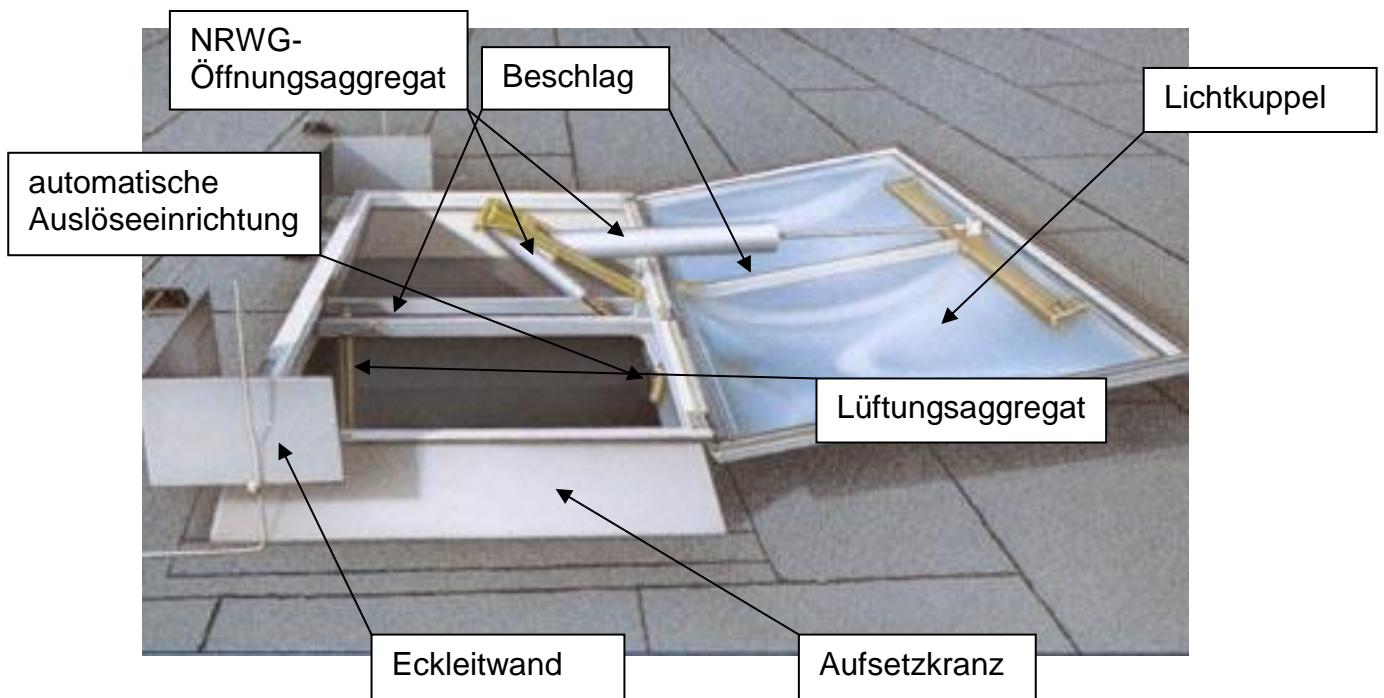
Bild 2: Beispielhafte Darstellung für ein in einer Lichtkuppel integriertes NRWG
